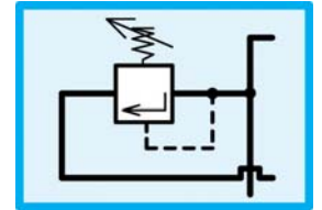
Valvola di massima Relief valve Max.Ventil
