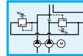
Pompa doppia con valvola disgiuntiva Two stage pump with pressure relief valve doppelte Pumpe mit Druckentlastungs-Ventil
